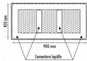
Obr.2. Lepenie zadnej strany styrcovej dosky
