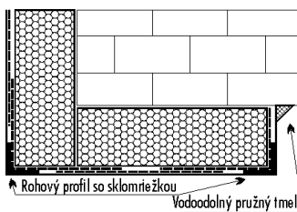
Obr.8. Vystruženie rohu a spôsob ukončenia zateplenia na rovnej fasáde s príznanou hranou
