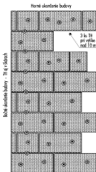
Obr.1. Ukladanie styrcových dosiek na väzbu a spôsob ich kovenia na fasáde
