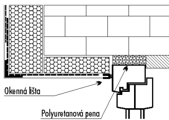
Obr.12. Zateplenie ostenia s použitím dilatanej okennnej lišty
