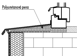
Obr.11. Zateplenie pri parapete purpenou
