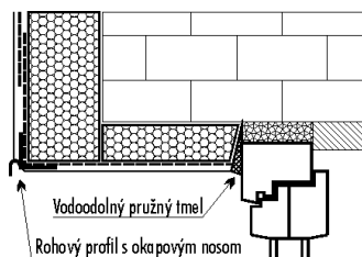
Obr.13. Zateplenie nadpražia s použitím okapového rohového profilu
