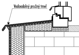
Obr.10. Zateplenie pri parapete
