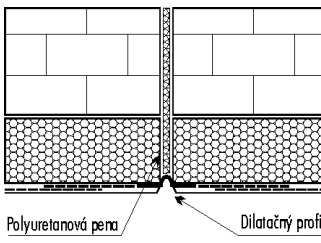
Obr.17. Priznanie dilatanej škáry pomocou dilatčného profilu
