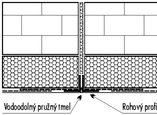
Obr.16. Priznanie dilatanej škáry pomocou dvoch rohových profilov
